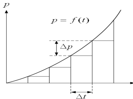
圖 1：連續函數之數位積分
